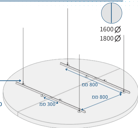
פרופיל T24
