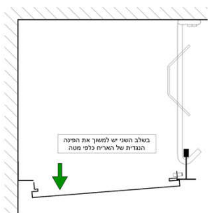
מצב 2 - תקרת X Lock 1:2
