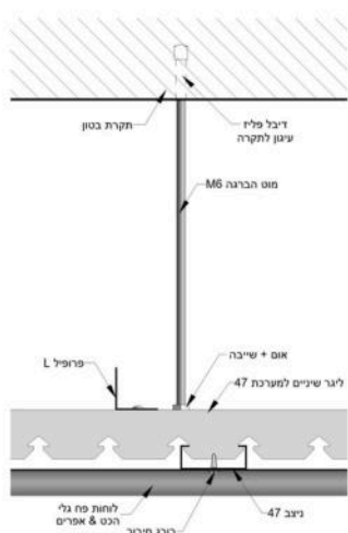
פרט 2 תקרה גלית 1 : 2
