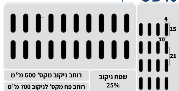
ניקוב אובלי 4X15 מ"מ OB40
