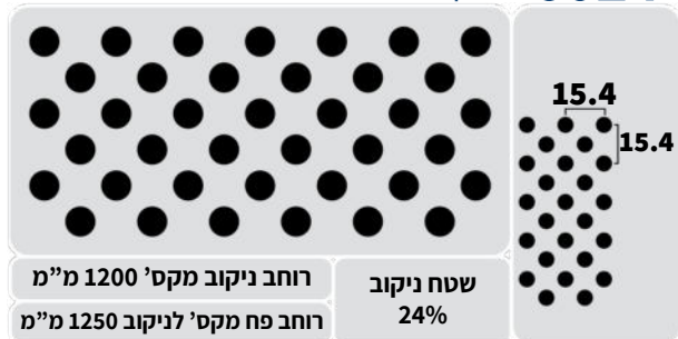
ניקוב עגול 6 מ"מ
