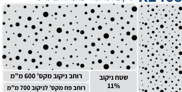
ניקוב רנדומלי 2X4X6X8 מ"מ R2468
