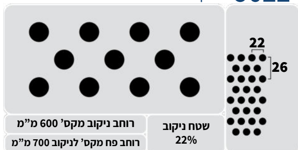
ניקוב עגול 9 מ"מ 9022
