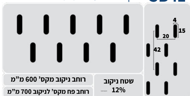
ניקוב אובלי 4X15 מ"מ SB41
