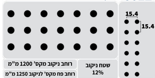
ניקוב עגול שורות ישרות 6 מ"מ
