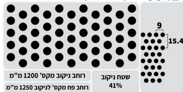
ניקוב עגול צפוף 6 מ"מ
