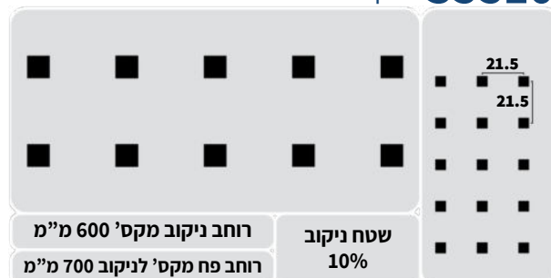
ניקוב מרובע 5.5X5.5 מ"מ S5510
