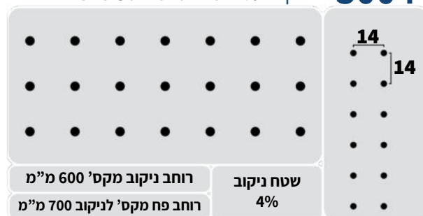
ניקוב עגול שורות ישרות 3 מ"מ
