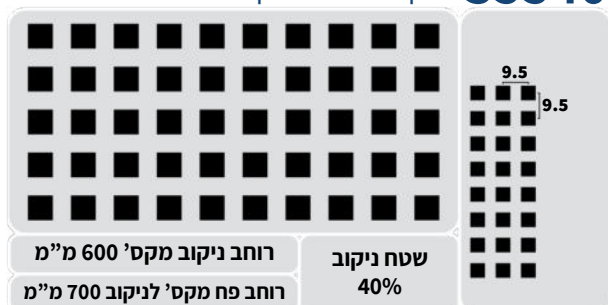
ניקוב מרובע צפוף 5.5X5.5 מ"מ S5540
