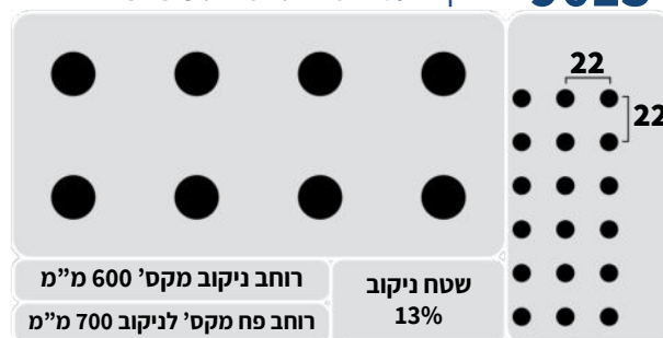
9013 ניקוב עגול שורות ישרות 9 מ"מ
