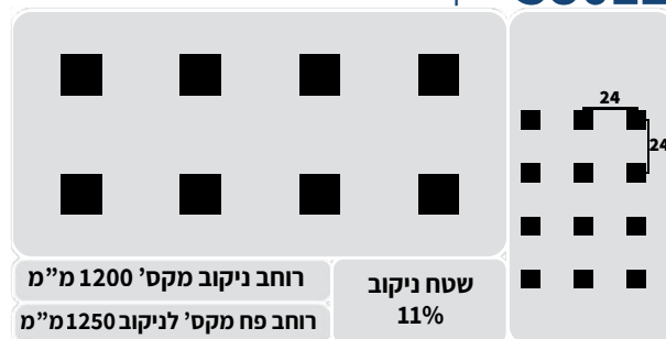
S8011 ניקוב מרובע 8X8 מ"מ
