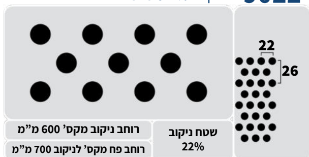
9022 ניקוב עגול 9 מ"מ
