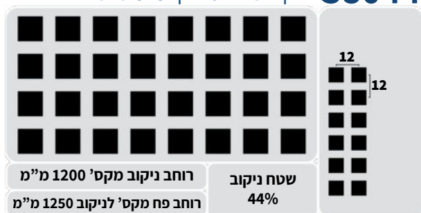
S8044 ניקוב מרובע צפוף 8X8 מ"מ
