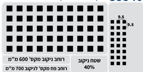
S5540 ניקוב מרובע צפוף 5.5X5.5 מ"מ
