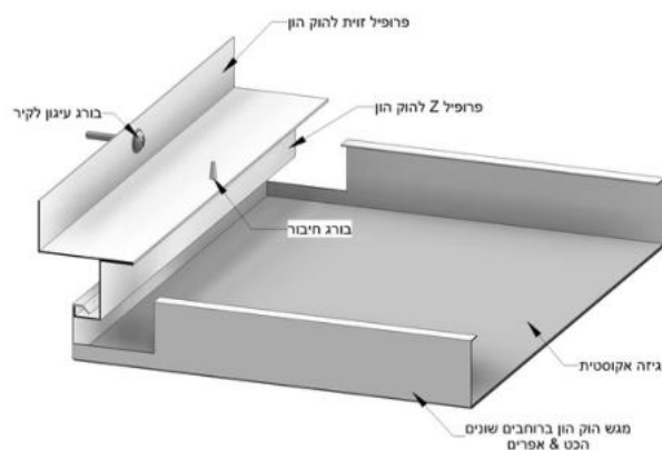
פרט תקרת הוק הון מסדרונות 1 : 2
