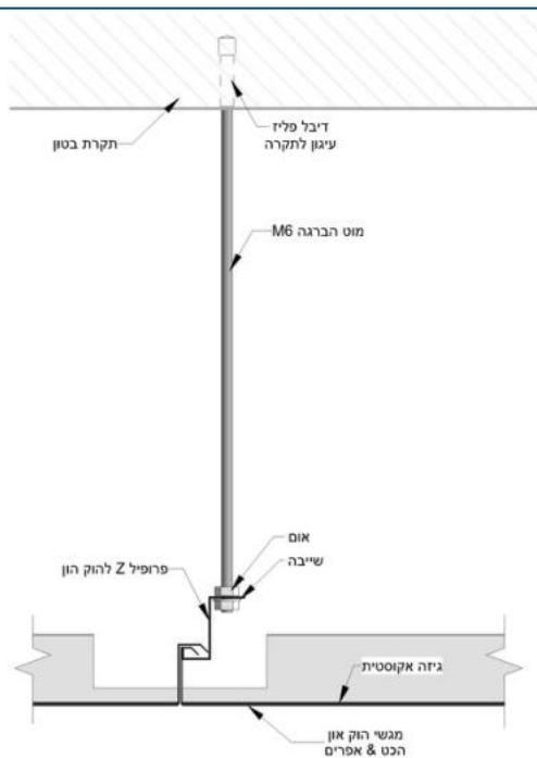
פרט תקרת הוק הון לחדרים 1 : 2
