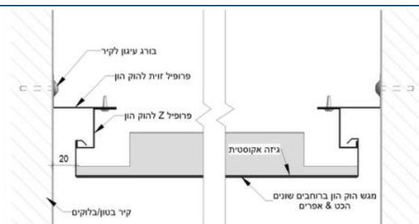
פרט תקרת הוק הון מסדרונות 1 : 2
