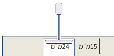
עומק שקיע 15 מ"מ
