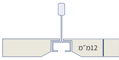
עומק שקיע 12 מ"מ
