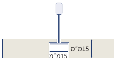
עומק שקיע 15 מ"מ + פזה
